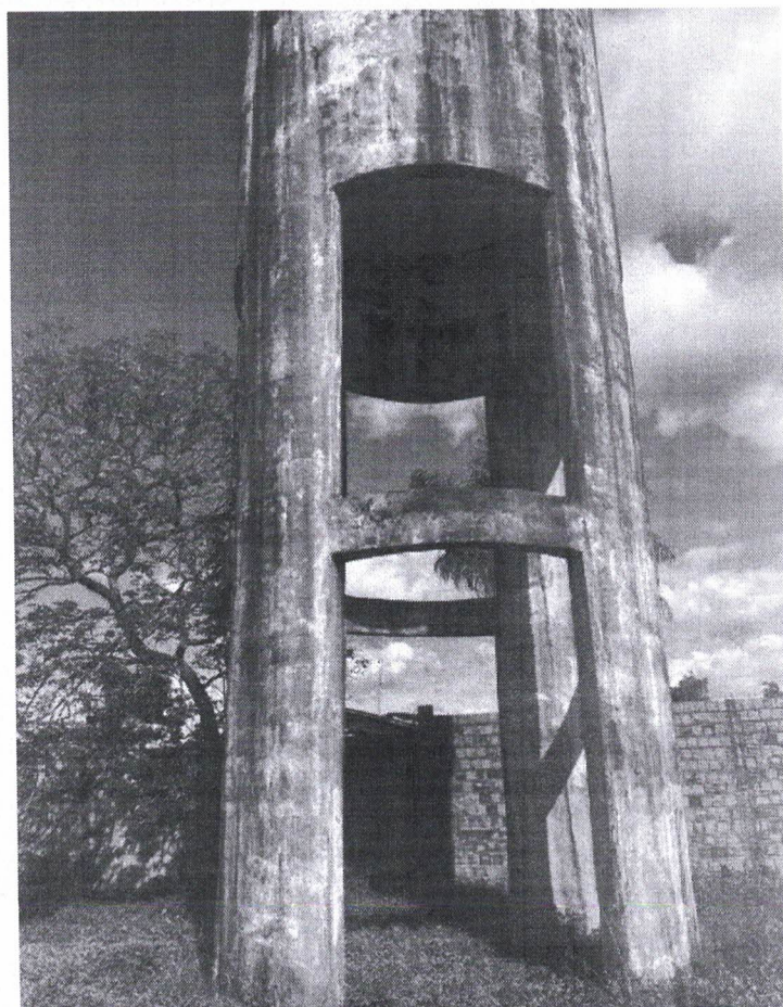
Reservatório existente com problemas estruturais e patologias.
