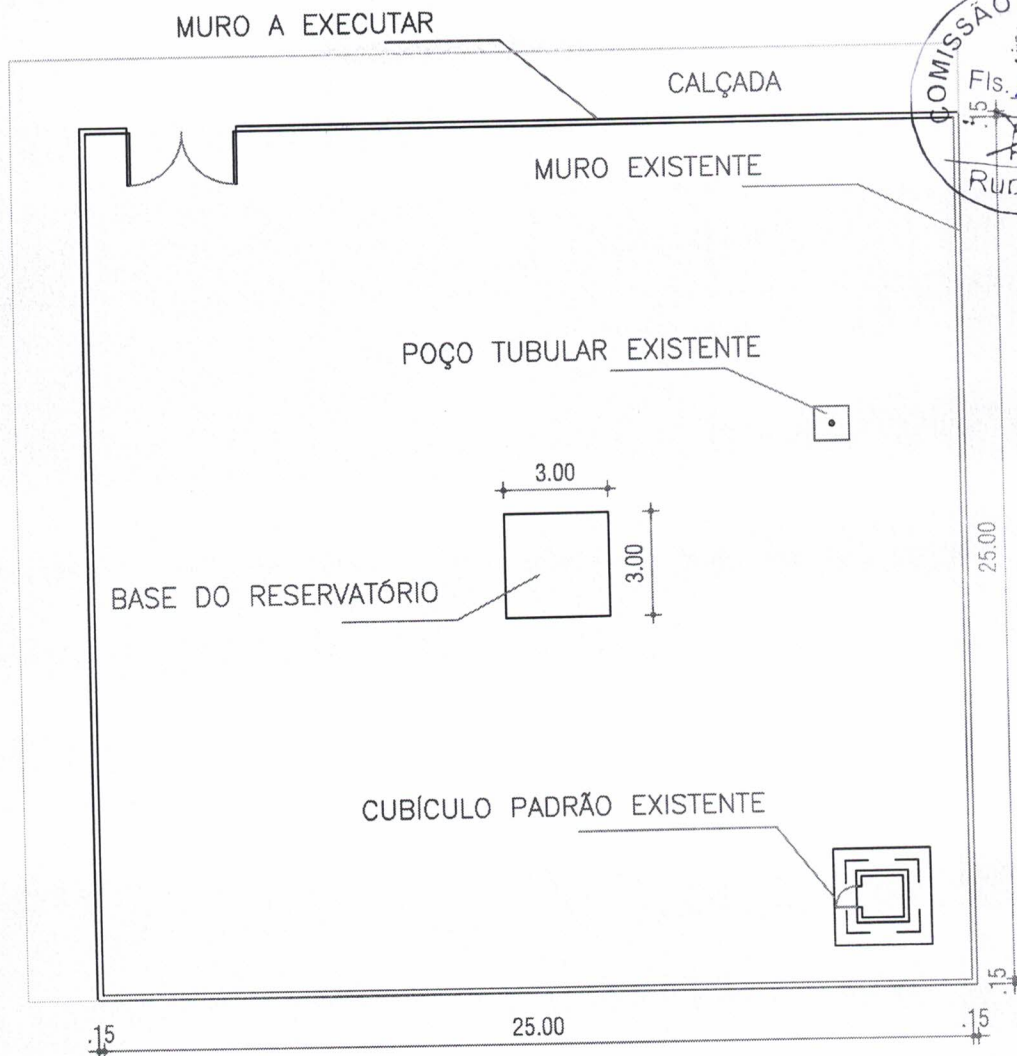
DETALHE DE IMPLANTAÇÃO ESCALA: 1:100
