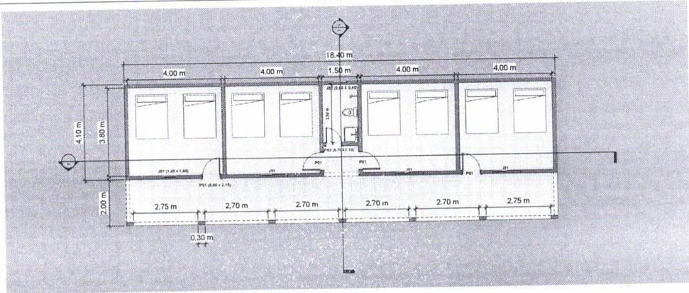
1 PLANTA BAIXA 1 : 50
