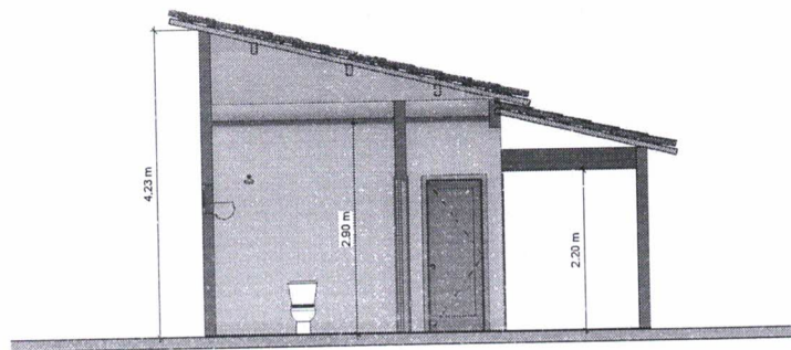
① Corte 1 1:25
